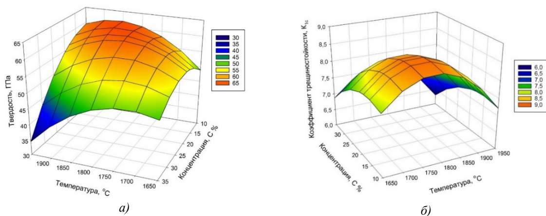
Рис. Зависимость твердости Y_{H_v} (a) и трещиностойкости Y_{K_{1c}} (б) от температуры и концентрации добавки УДА-порошка при постоянном давлении ( P = 6,5 ГПа)
