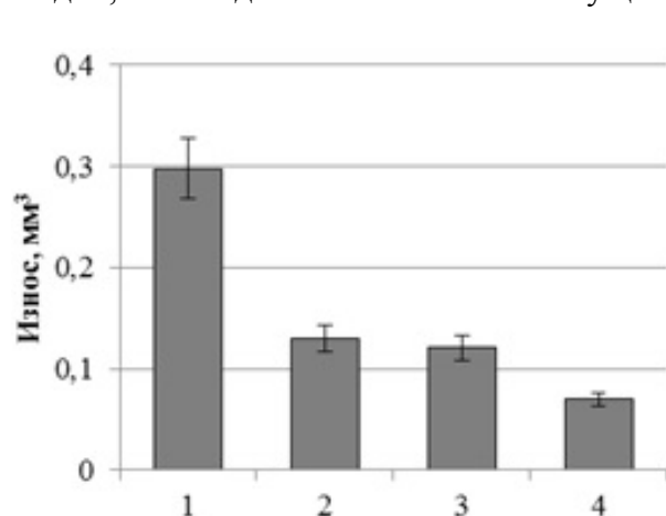
Рис. Величина объемного износа (мм³) ПЭЭК (1), СВМПЭ (3) и композитов ПЭЭК + 1 вес.% УНТ (2), СВМПЭ + 1 вес.% УНВ (4) при сухом трении скольжения; нагрузка 60 Н, путь трения 1080 м
