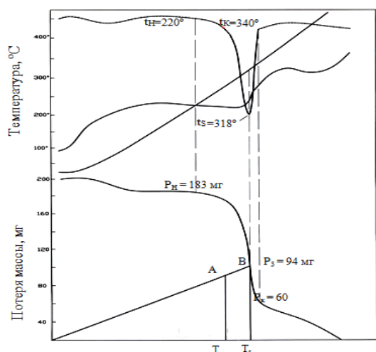
Рис. 2. Девиватограмма карбонизации вязкого волокна после ТВО
