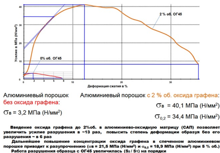
Рис. 1. Влияние оксида графена на прочность спечённых алюминиевых порошков
