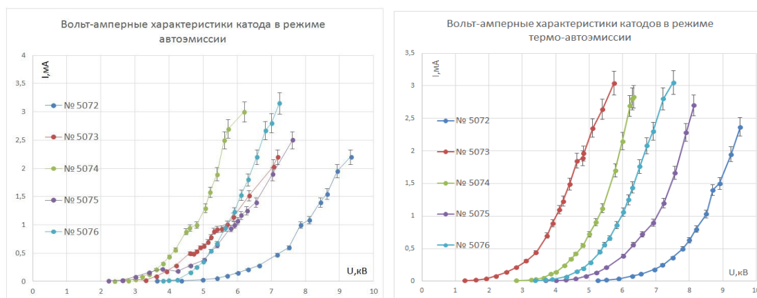
Рис. Вольт-амперные характеристики катодов в режиме автоэмиссии (20 °C) и в режиме термо-автоэмиссии (800 °C)
