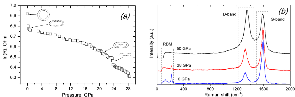
Рис. 1. Барическая зависимость электросопротивления двустенных нанотрубок (a). Спектры КР двустенных углеродных нанотрубок (b)
