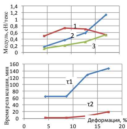
Рис. 2. Изменение модулей стабильной сетки (1) и релаксационных компонент (2), (3), времен релаксации \tau_1 , \tau_2 (b) при деформации.
