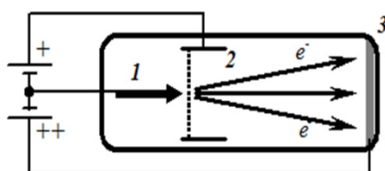
Рис. Схематическая конструкция катодолюминесцентной пальчиковой лампы
