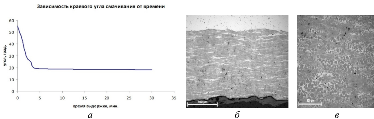
Рис. Зависимость краевого угла смачивания от времени выдержки ( а ) и структура граффлекса при времени выдержки 2 мин ( б ) и силицированного граффлекса ( в )
