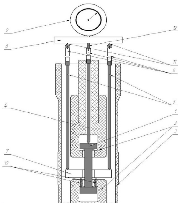
Рис. 1. Схематическое изображение дилатометрической системы измерения деформации: 1 – испытываемый образец, 2 – графитовые (либо УУКМ) захваты, 3 – графитовый нагреватель, 4 – центральный графитовый стержень, 5 – боковые графитовые стержни, 6 – кварцевые стержни, 7 – графитовое коромысло, 8 – платформа, 9 – измерительная головка, 10 – иглообразные стержни, 11 – стальные наконечники, 12 – подвижный шток индикатора часового типа
