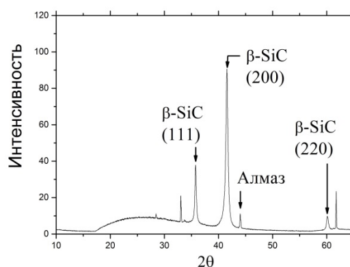
Рис. 2. Дифрактограмма композита « \beta -SiC-алмаз»
