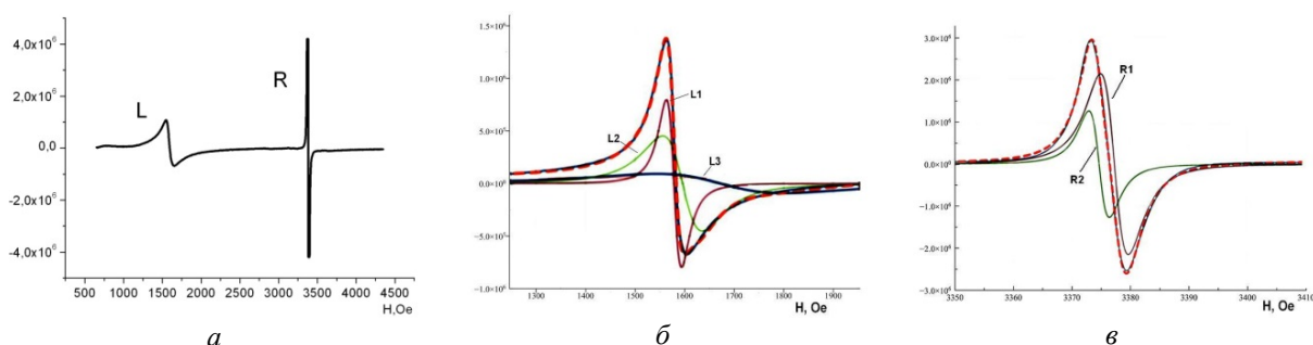
Рис. Спектр ЭМР (Канско-Ачинский бурый уголь, 300 К):
