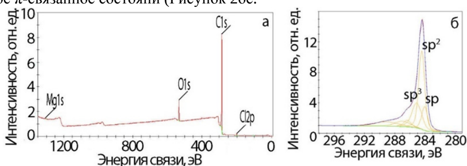
Рис.2. (а) Обзорный рентгеновский фотоэлектронный спектр, (б) спектр высокого разрешения C1s ИСУП, синтезированной на магнии
