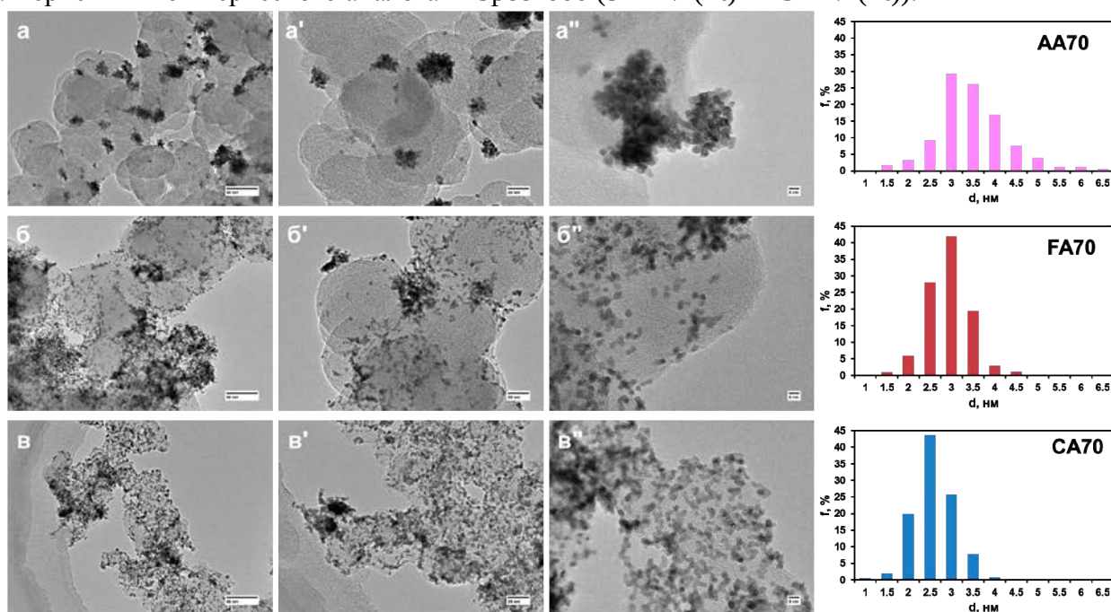
Рисунок 2. Микрофотографии ПЭМ катализаторов Pt/C, синтезированных в углеродных суспензиях при 70 °С с использованием различных восстановителей: аскорбиновая кислота (а, а', а''), муравьиная кислота (б, б', б''), лимонная кислота (в, в', в'')
