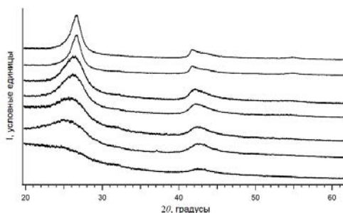
Рис. 1. Дифрактограммы образцов гексагонального нитрида демонстрируют, что полученные частицы имеют различный размер.
