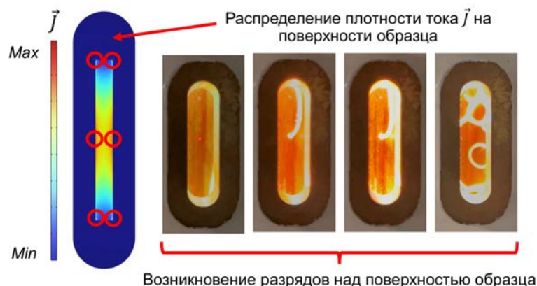
Рис. 1. Возникновение разрядов над поверхностью образца графита (слева – расчетные данные по распределению плотности тока с выделенными областями максимальных значений J ; справа – разряды во время процесса модификации, фото).
