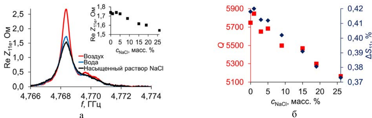
Рис. 2. Изменение параметров сенсора вследствие нанесения водных растворов NaCl различной концентрации для обертона на частоте 4,8 ГГц: изменения амплитуды и формы сигнала (а); зависимости добротности и коэффициента отражения сенсора от концентрации раствора NaCl (б)
