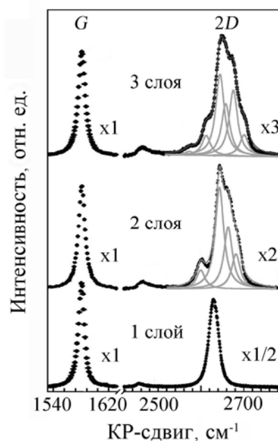
Рис. 2. Экспериментальные G и 2D полосы спектров КР одно- и несколькослойных графенов (точечные линии) и аппроксимация 2D пиков лоренцианами (серые линии). При оформлении рисунка были использованы данные из [3].
