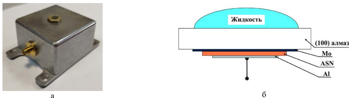
Рис. 1. Корпусированный СВЧ акустоэлектронный сенсор (а) и схема чувствительного элемента (б).
