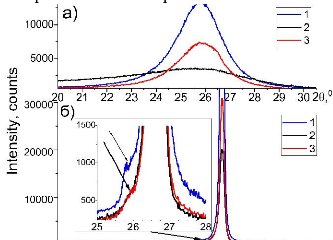
Рис. 1 Участок рентгенограммы с рефлексом 002: 1 – игольчатого кокса; 2 – закоксованный пек; 3 – образца АМ2: а) до графитации; б) после графитации.
