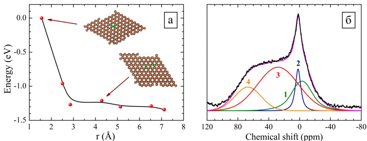
Рис. 2. (а) - Энергия кластера графена как функция расстояния между двумя атомами бора; (б) - ЯМР ^{11}B спектр алмаза с содержанием бора \sim 1\% (записан при вращении под магическим углом с частотой 20 кГц)
