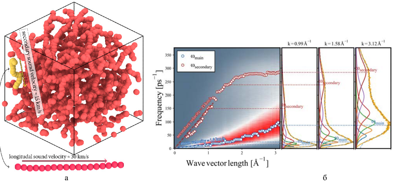
Рис. 1. Визуализация жидкого углерода при T = 5000 К, \rho = 0,5 г/см 3 (а); цветная 2D-тепловая карта спектров возбуждения жидкого углерода при T=6000 К, \rho = 0,5 г/см 3 с точками, обозначающими пики. Справа приведены подробные спектры возбуждения CL(\omega) (в условных единицах) для различных длин волнового вектора (б)
